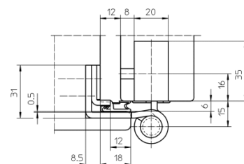
фальц 18 мм (головная часть уплотнителя 12 мм)
