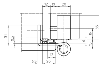
фальц 20 мм (головная часть уплотнителя 12 мм)
