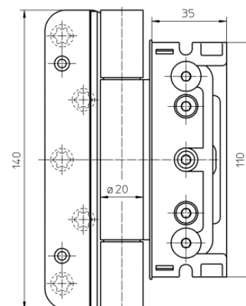
Вид спереди 18 мм
